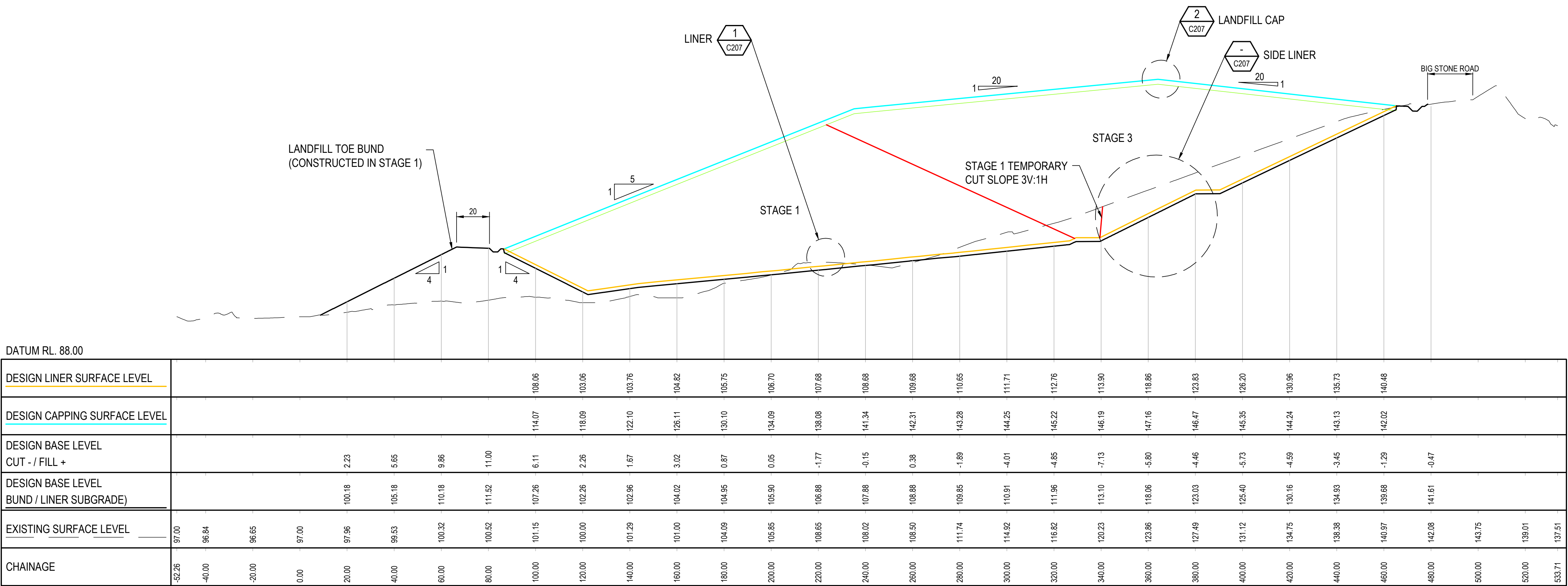
LONGITUDINAL SECTION - SECTION B (LANDFILL)
